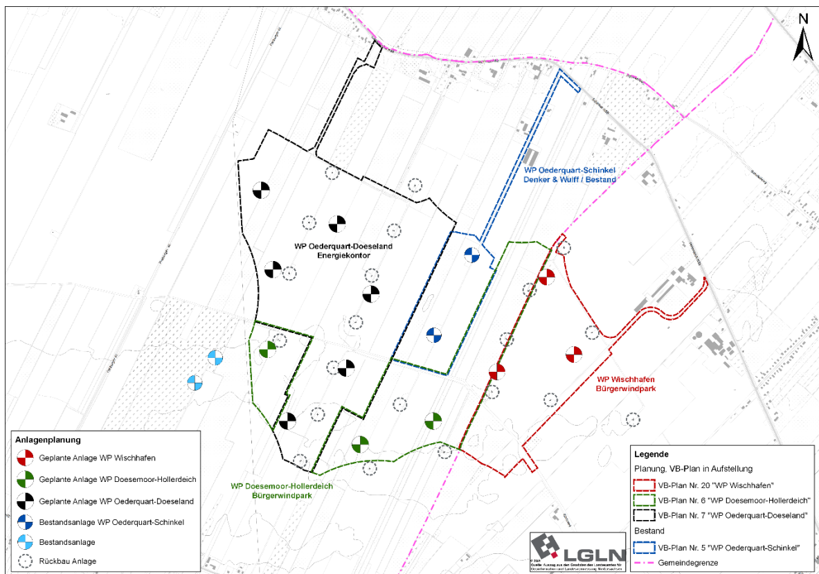
Abbildung 2: Lage der drei geplanten WEA (rote Kreise) im Geltungsbereich zum vorhabenbezogenen B-Plan Nr. 20 „Windpark Wischhafen“ (rot gestrichelt) im Verhältnis zu den weiteren vorhabenbezogenen B-Plänen der benachbarten Windparks (grün, schwarz und blau gestrichelt). Die Altanlagen sind als hellgrau gepunktete Kreise dargestellt.
