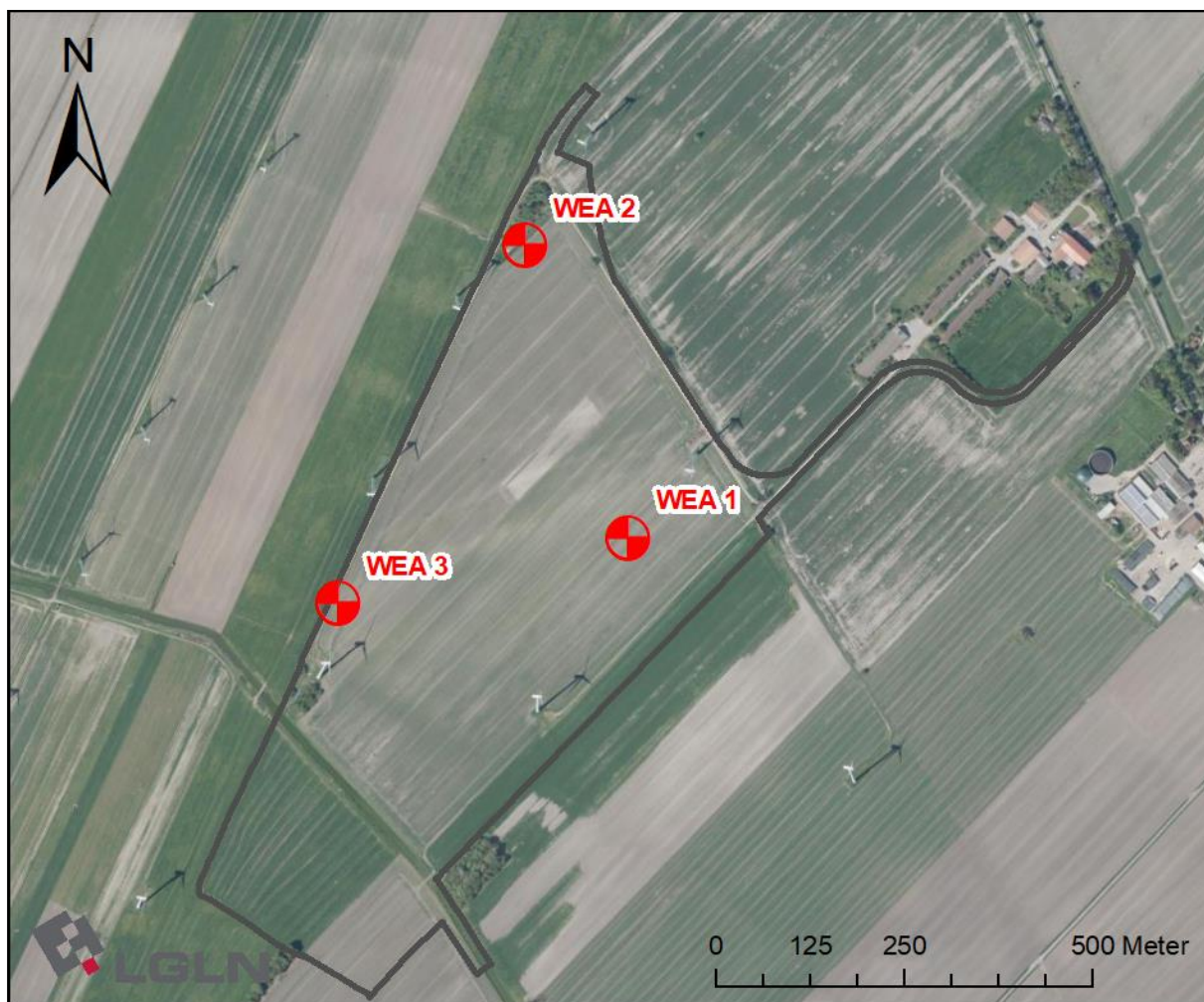
Abbildung 4: Lage der geplanten WEA (roter Kreis) im Plangebiet (dunkelgraue Linie). M 1 : 10.000.
